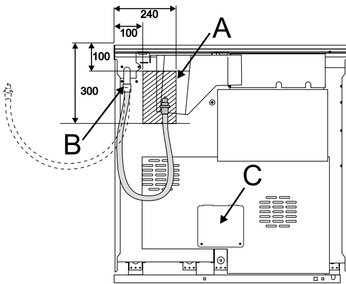
Vue arrière
