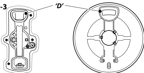
A – Chapeau de brûleur interne, B – Chapeau de brûleur externe, C – Tête de brûleur interne, D – Tête de brûleur externe, E – Socle de brûleur de Wok
