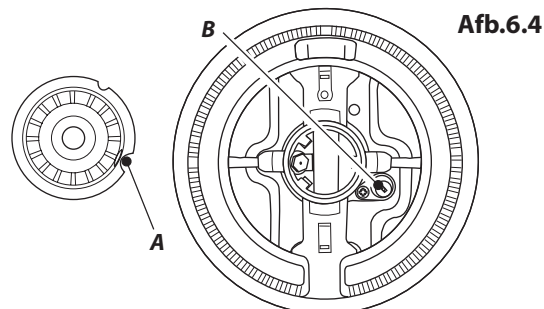
A – Elektrode-inkeping, B – Ontstekings elektrode
