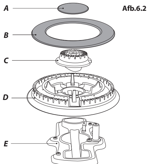
A – Binnenbranderkap, B – Buitenbranderkap, C – Binnenbranderkop, D – Buitenbranderkop, E – Wokbranderbasis
